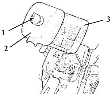
KRAFTSTOFF-FILTER Bild 1
